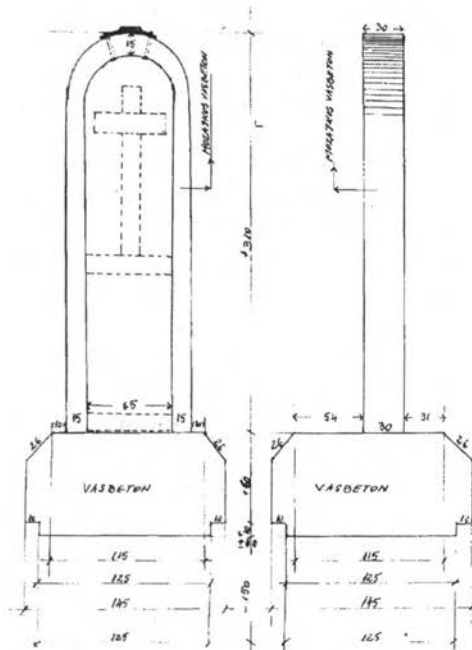
Az emlékmű méretei
