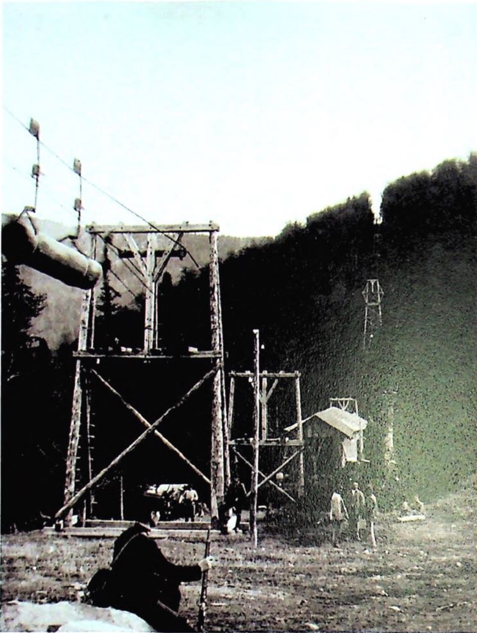
Fát szállító sodrony 1905-ben
