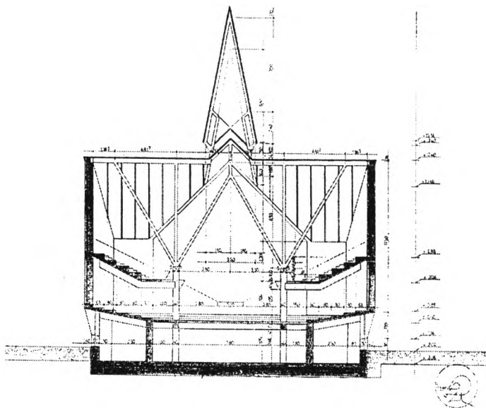
Keresztmetszet
