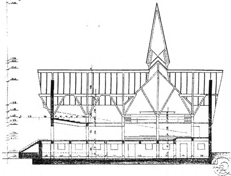
Hosszmetszet
