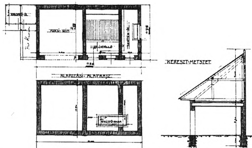
A melléképület alapozási rajza, alaprajza és keresztmetszete
