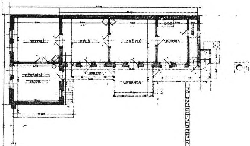
A földszint alaprajza
