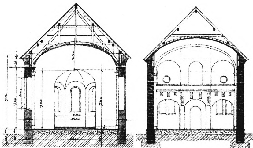
Az oltár és a kórus felőli metszetek
