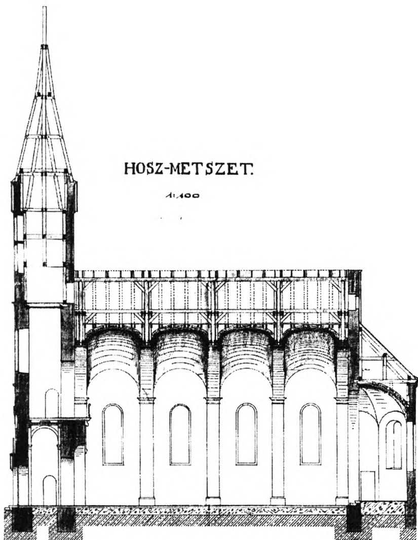
A csernátfalusi római katolikus templom hosszmetsete
