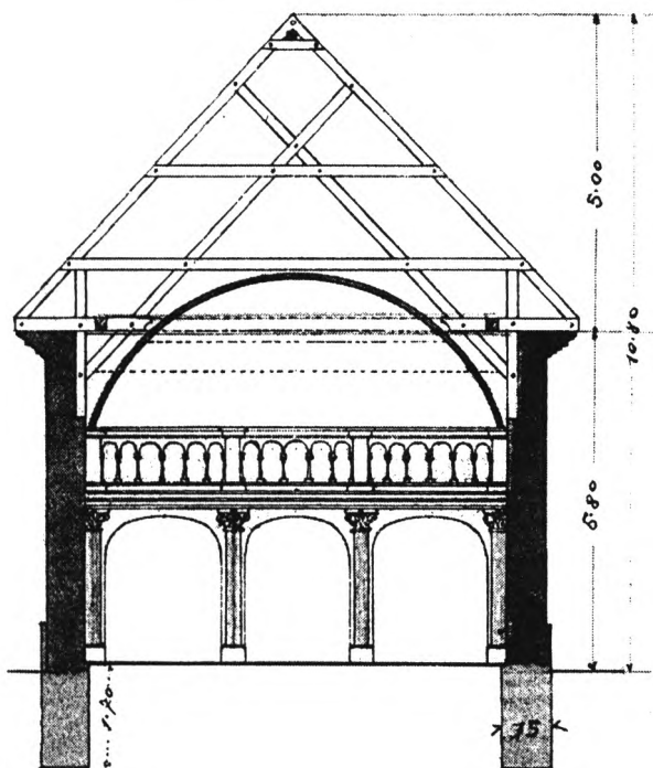
A kórus felőli metszet
