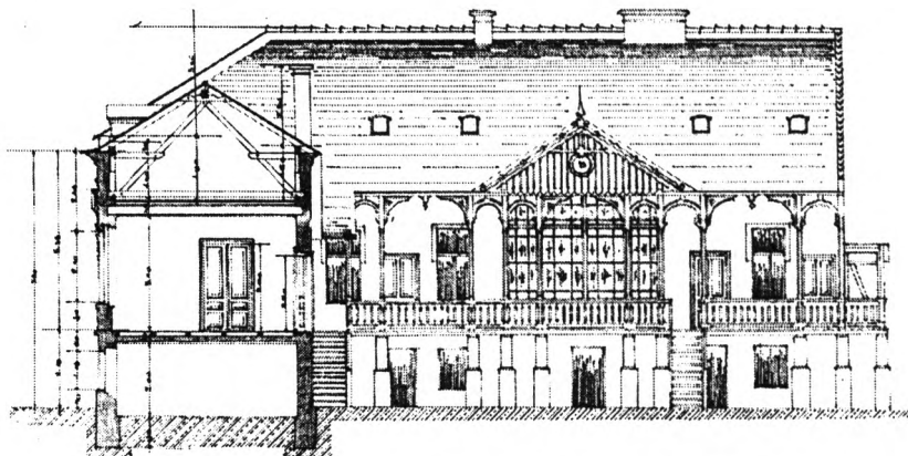
A plébánia keresztmetszete és udvari nézete
