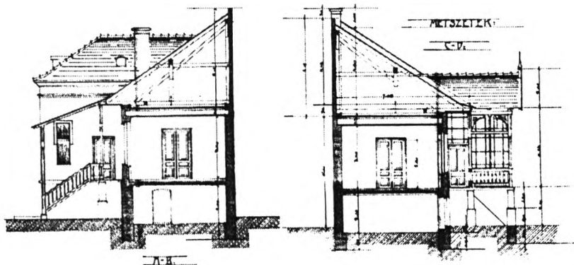
A plébániaépület különféle metszetei
